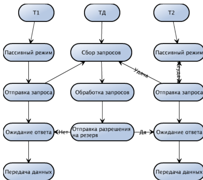
Рис. 1.3 Метод множественного доступа DAMA
